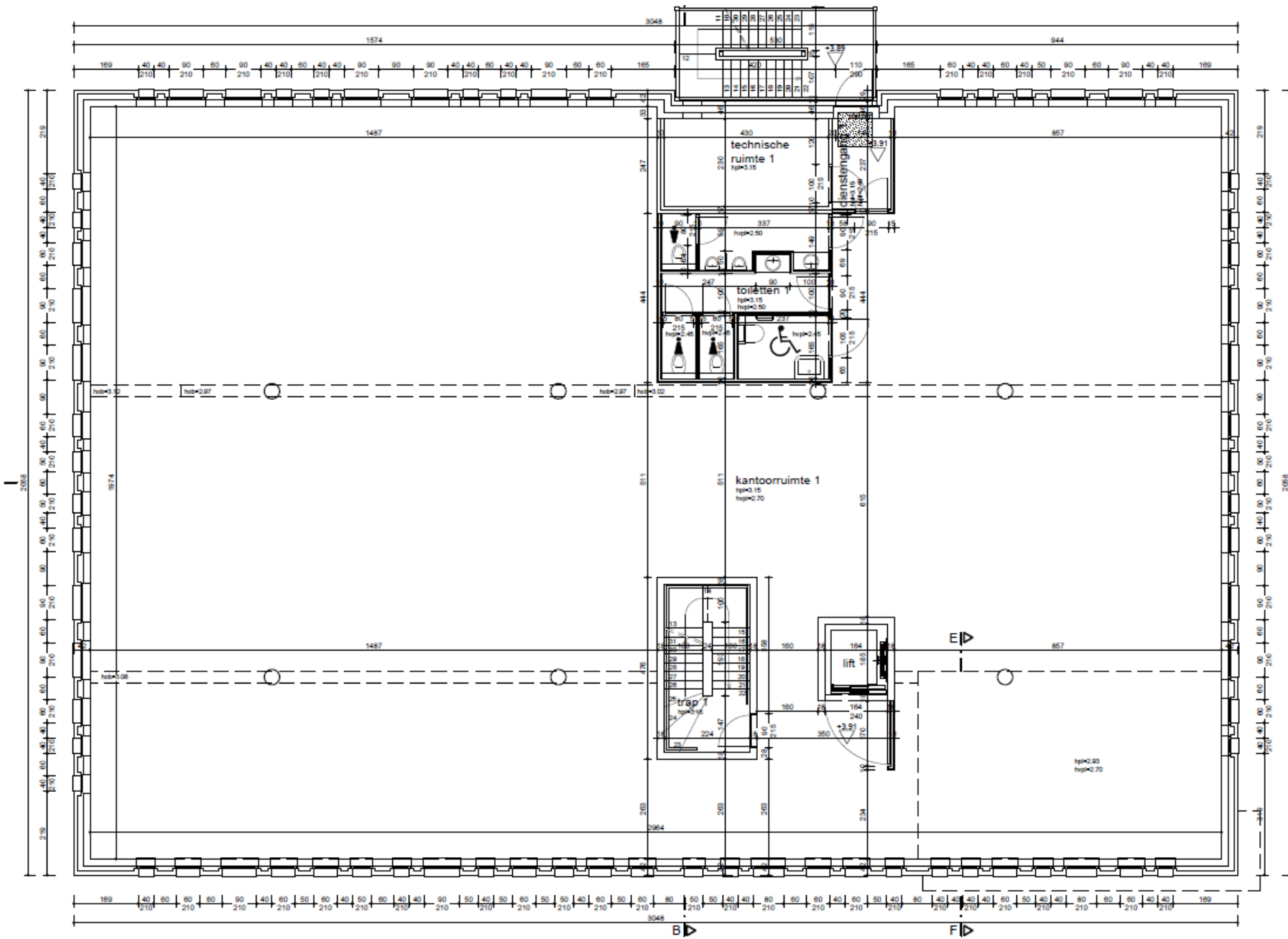
EERSTE ETAGE
