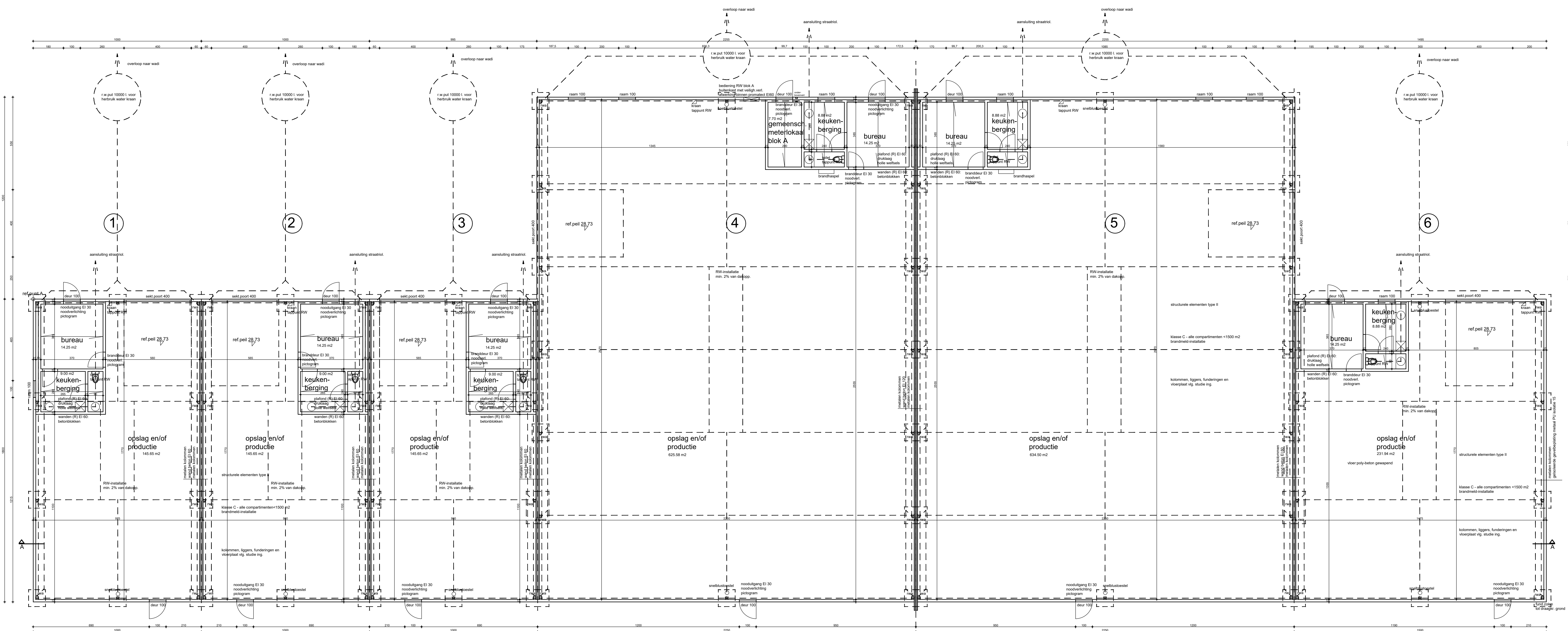
niveau (-01) 00 A nieuw 1/100
